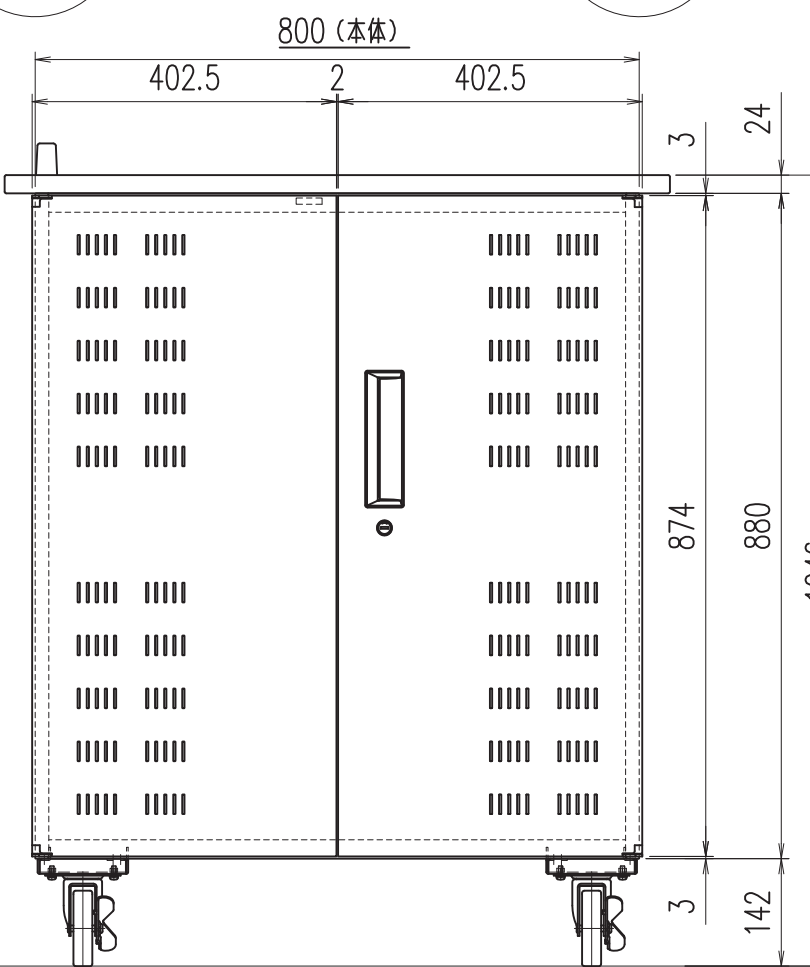
正面図
