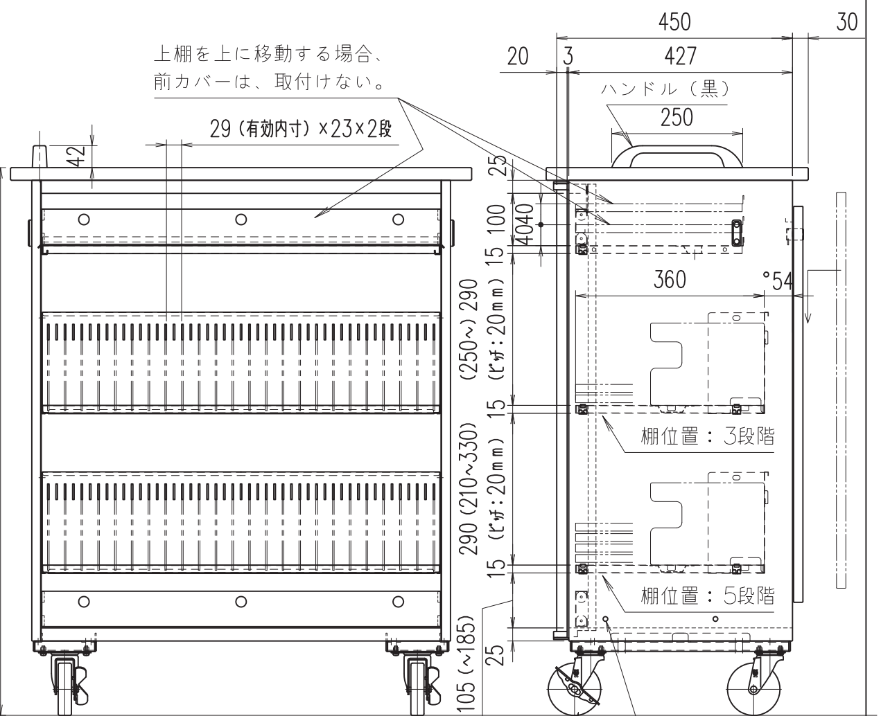
扉を外した状態の正面図
