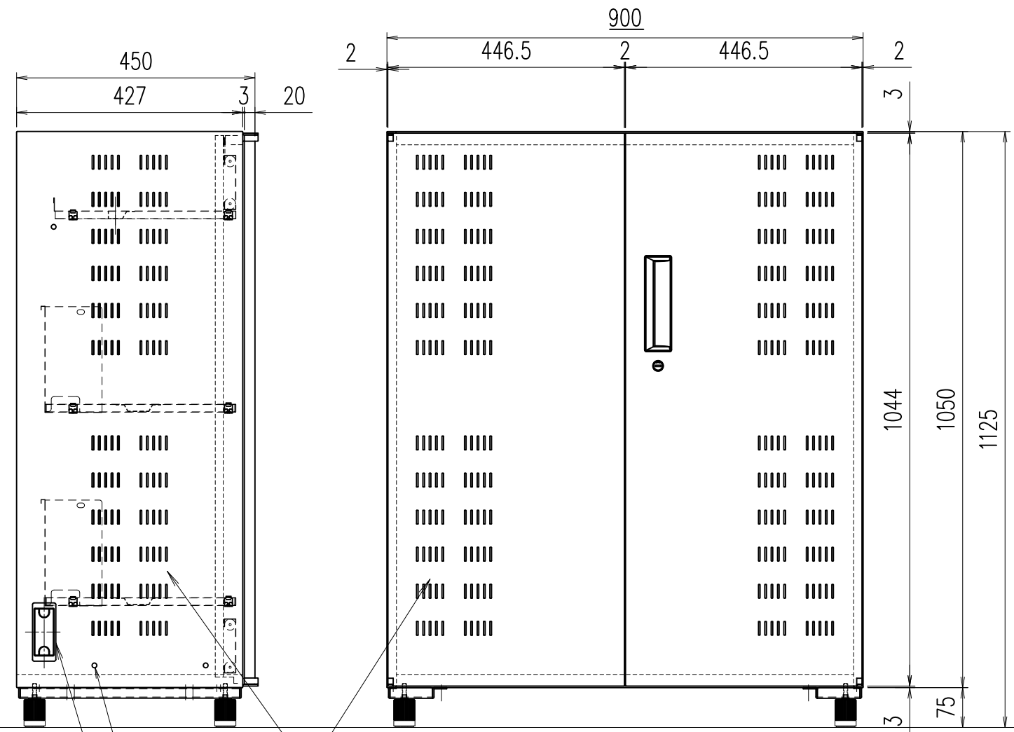
正面図
