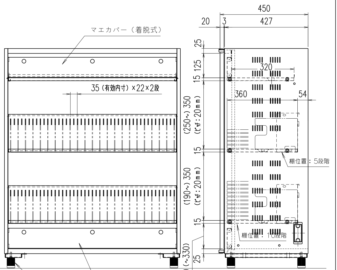
扉を外した状態の正面図
