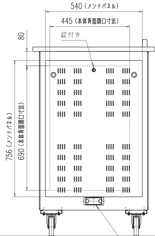
背面図
