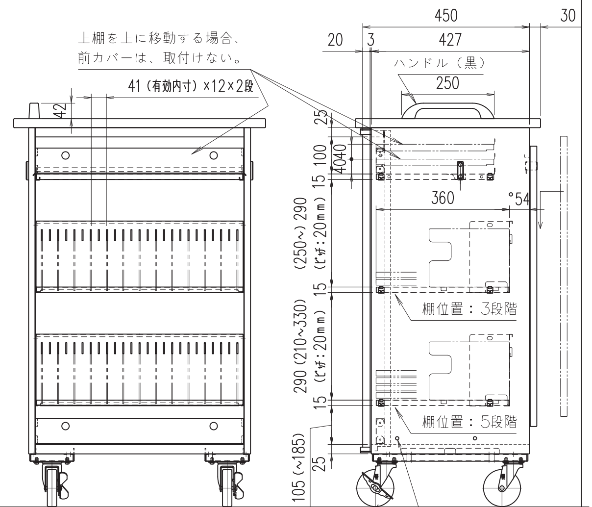
扉を外した状態の正面図
