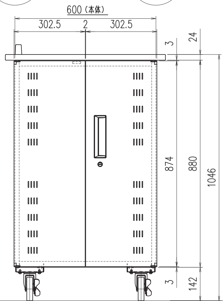
正面図
